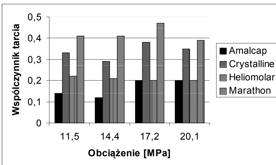
Rys.2. Opory tarcia w funkcji obciążenia
