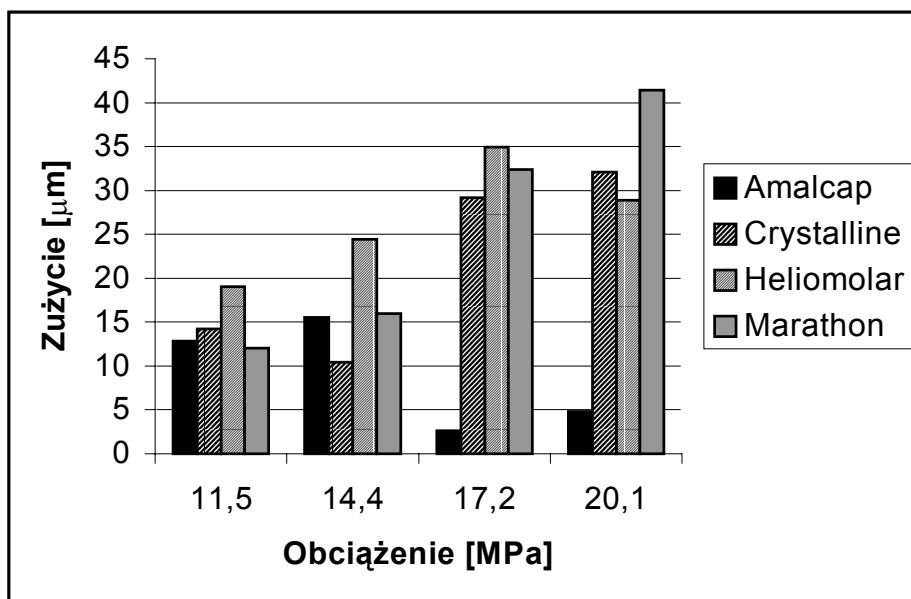
Rys.1 . Zużycie tribologiczne badanych materiałów
